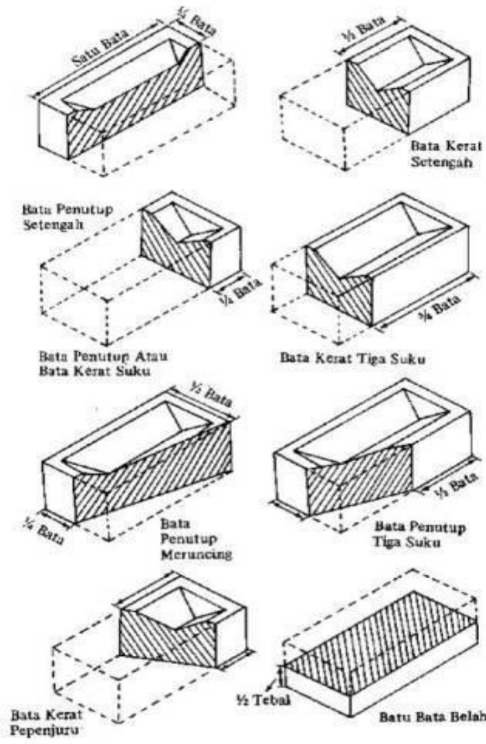
Fotongan batu bata
