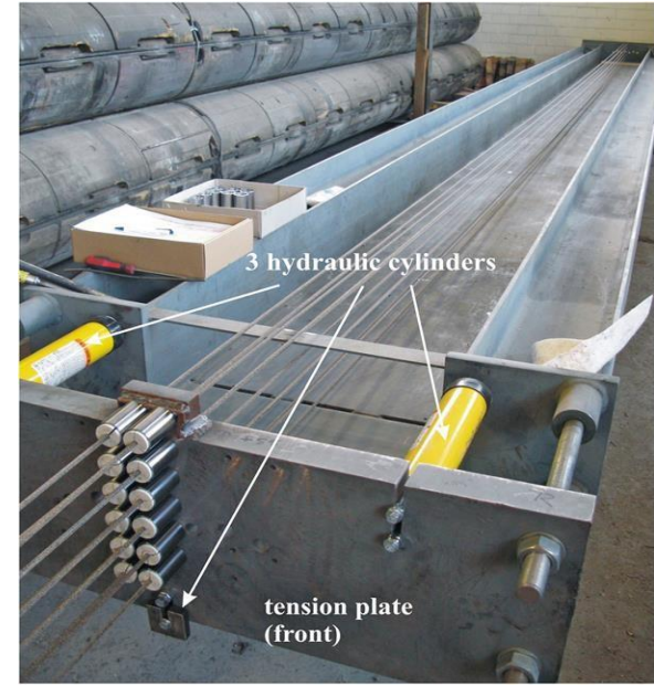
الشد السابق pre tensioning
